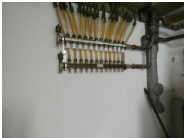
Fußbodenheizung
